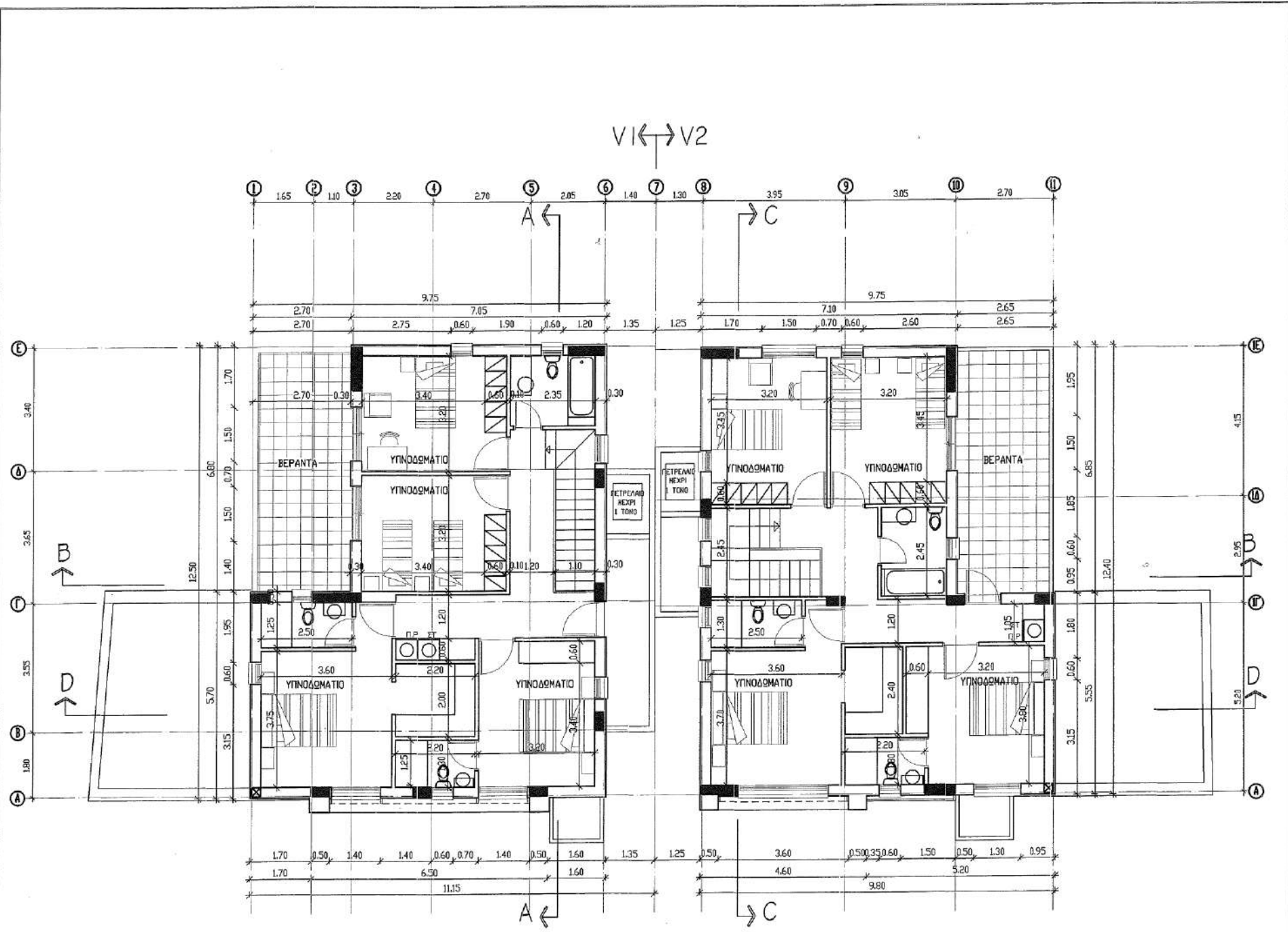
ΚΑΤΩΦΗ ΟΡΟΦΟΥ ΚΛΙΜΑΚΑ 1:100
