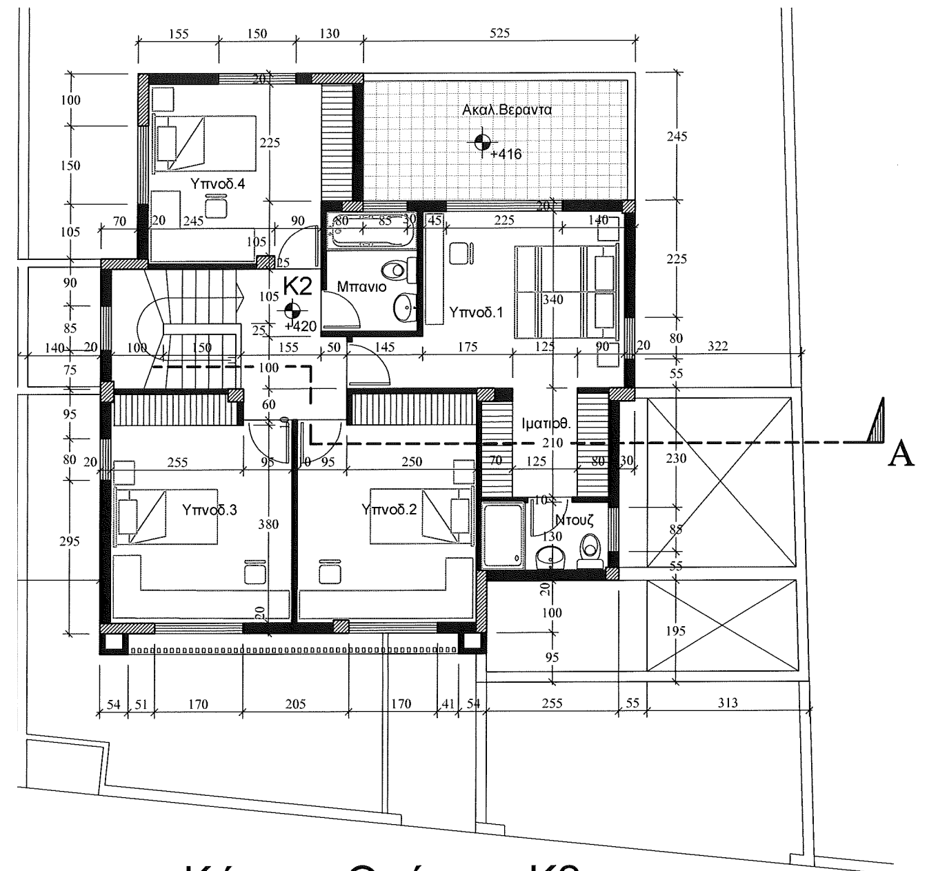
Κάτοψη Ορόφου Κ2
