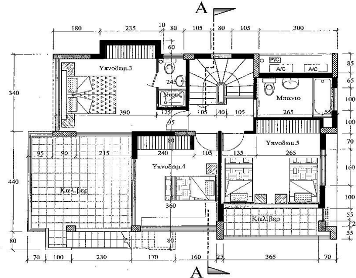
Κατοψη Οροφου
