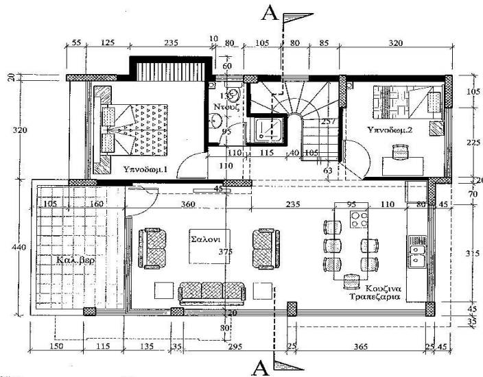
Κατοψη Ισογειου
