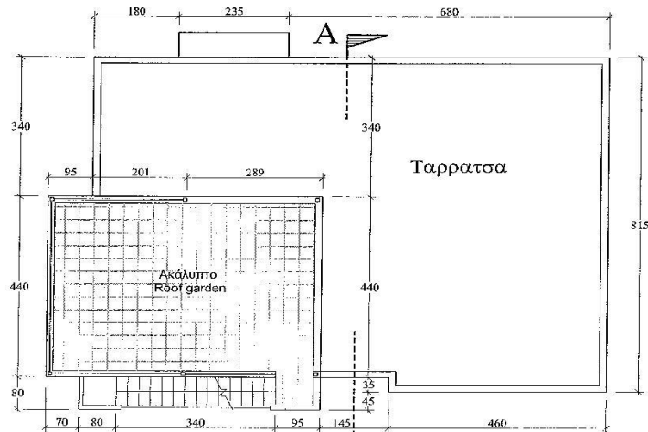
Ανωψη
