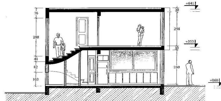
Τομη Α-Α
