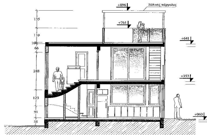
Τομη Α-Α
