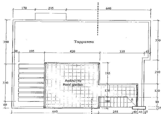
Ανωψη
