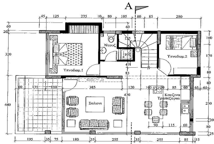
Κατοψη Ισογειου
