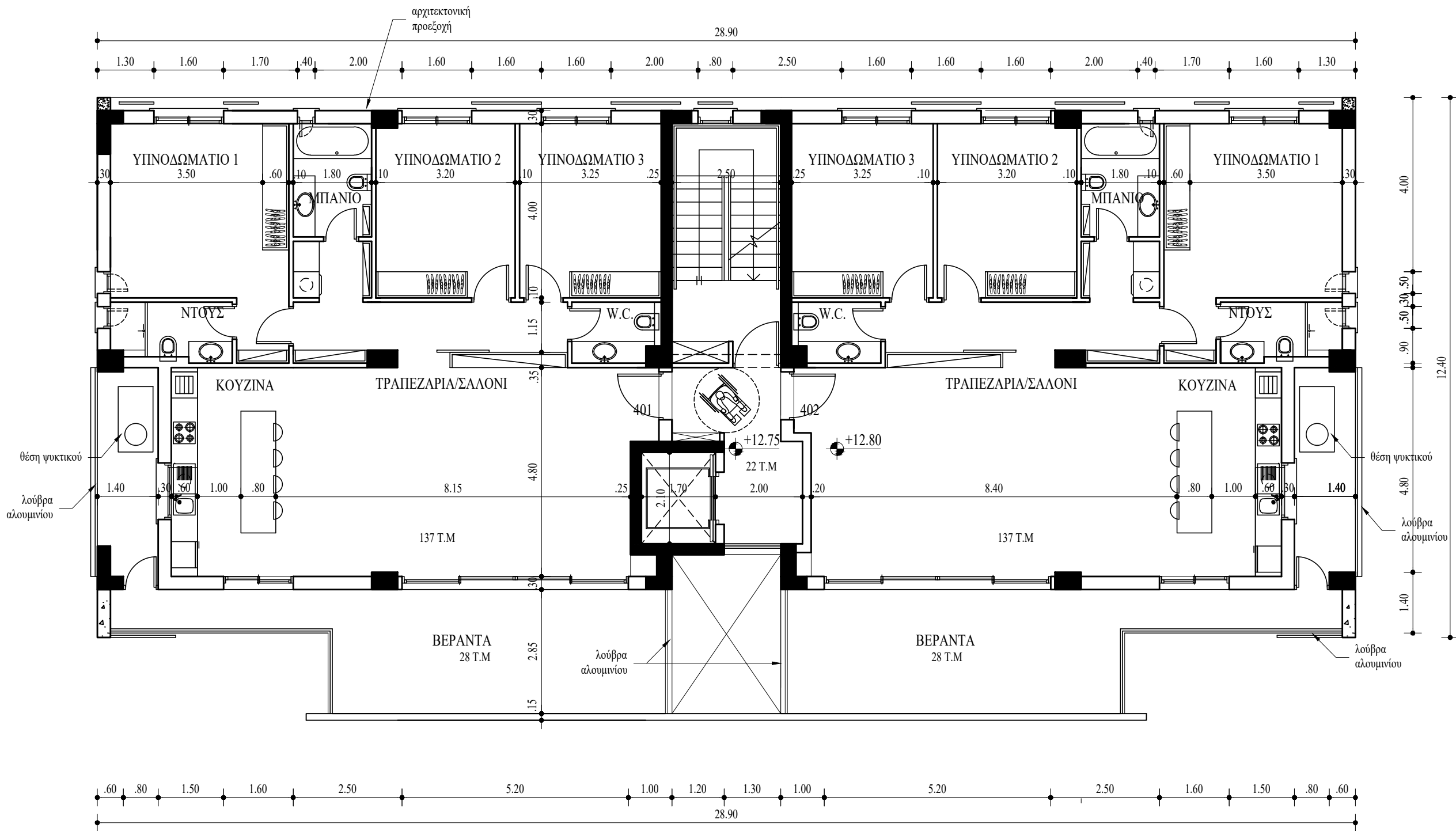
ΚΑΤΟΨΗ 4ου ΟΡΟΦΟΥ
